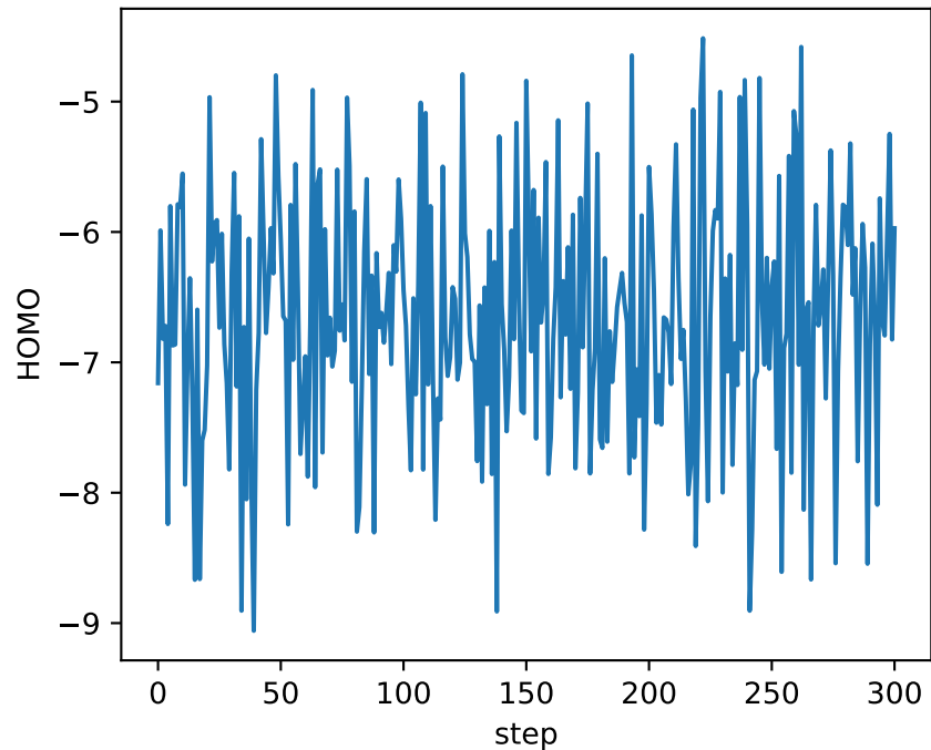
HOMO - evolution
